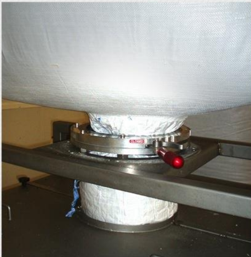
Задвижка 12" (305мм) работает на разгрузке биг-бэга
