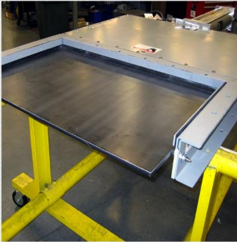
Задвижка 610мм x 965мм установлена в системе вибропитателя для дозирования потока угля
