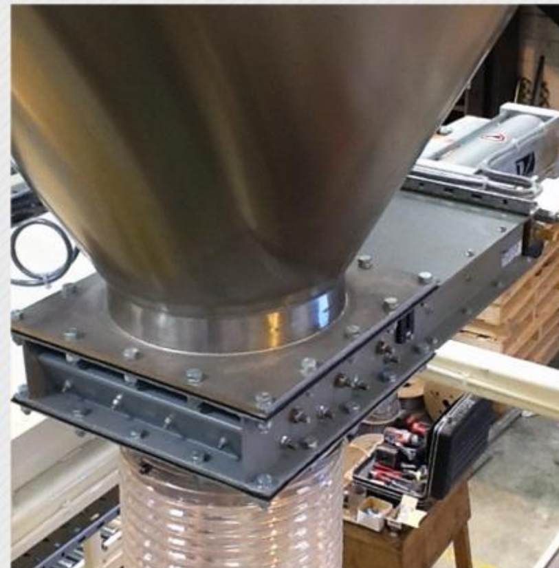
Задвижка 10" (254мм) работает с шлаком
